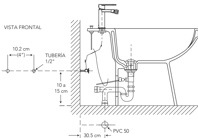
GRÁFICO REFERENCIAL DE INSTALACIÓN
